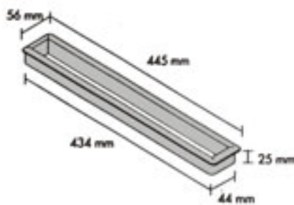
PASSE PAPIER PAPER GUIDE
