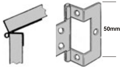
CHARNIÈRE RASÉE POUR PANNEAU 5/8" OU 11/16" FLUSH HINGE FOR 5/8" OR 11/16" PANEL
