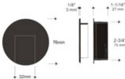
PASSE-FILS PLASTIQUE PLASTIC GROMMET
