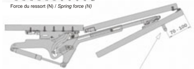
Système pour portes en bois / Wood door system
