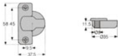
COIN MORT / BLIND CORNER
