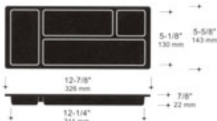
AUGET À CRAYONS PENCIL TRAY
