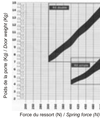
Systèmes pour portes PracticAL Door systems
