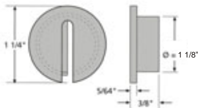
PASSE-FILS PLASTIQUE PLASTIC GROMMETS
